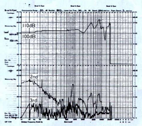
●SR-X/MK3Pro.周波数・歪特性
