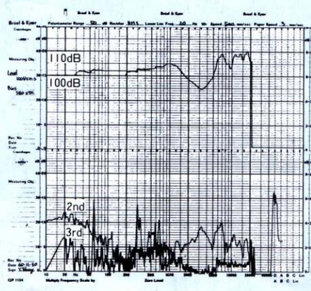
●SR-αPro.周波数・歪特性
